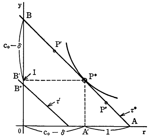
図・7 \theta=1 の場合
