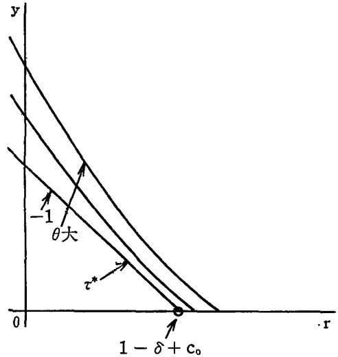
図・5 \theta \geq 1 のケース
